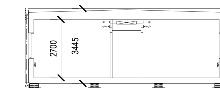
SNITT A-A 1:100
