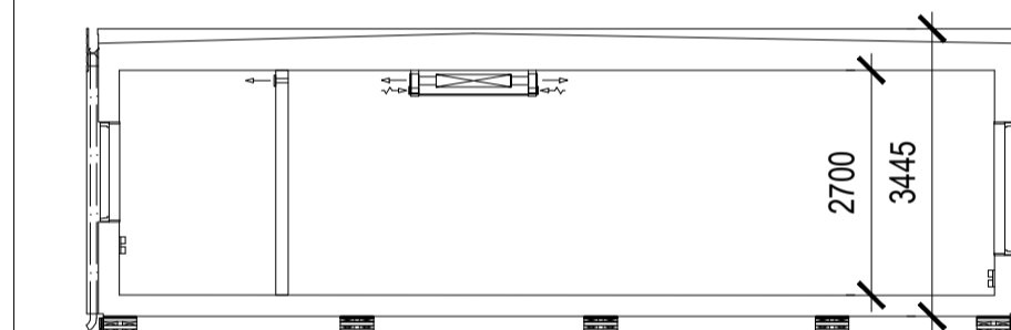
SNITT A-A 1:100
