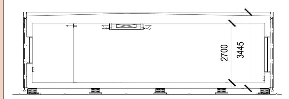
SNITT A-A 1:100
