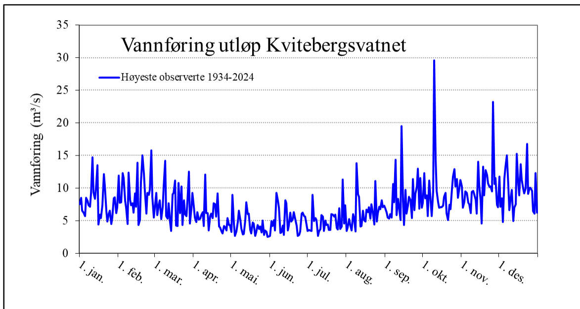
Figur 3. Plott som viser høyeste beregnede vannføring for hver dato gjennom året (døgndata) for vannføring i utløpet av Kvitebergsvatnet. Dette representerer ikke ett spesielt år, men viser de høyeste vannføringene per dato basert på hele den 90 år lange observasjonsserien fra 1934 til og med 2024 fra referansestasjon 55.4 Røykenes i Osvassdraget.
