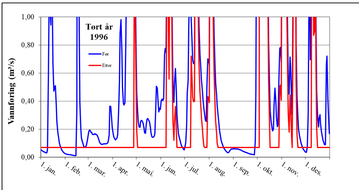
Figur 5. Plott som viser vannføringsvariasjoner ved utløp av Kvitebergsvatnet i et tørt år (1996) før (blå) og etter omsøkt uttak av 270 \text{ l/s} (rød) med slipp av minstevannføring på 70 \text{ l/s} . Oppfylling av nedtappet magasin er hensyntatt i figuren. For best mulig oppløsning, er bare vannføringer under 1 \text{ m}^3/\text{s} vist. Tallene er tilpasset fra referansestasjon 55.4 Røykenes i Osvassdraget.
