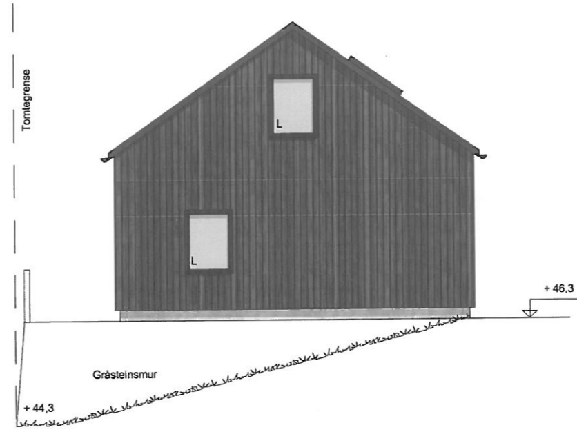
Fasade Øst
