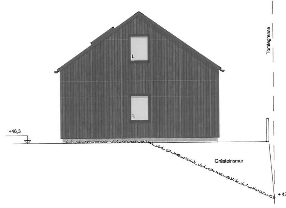
Fasade Vest
