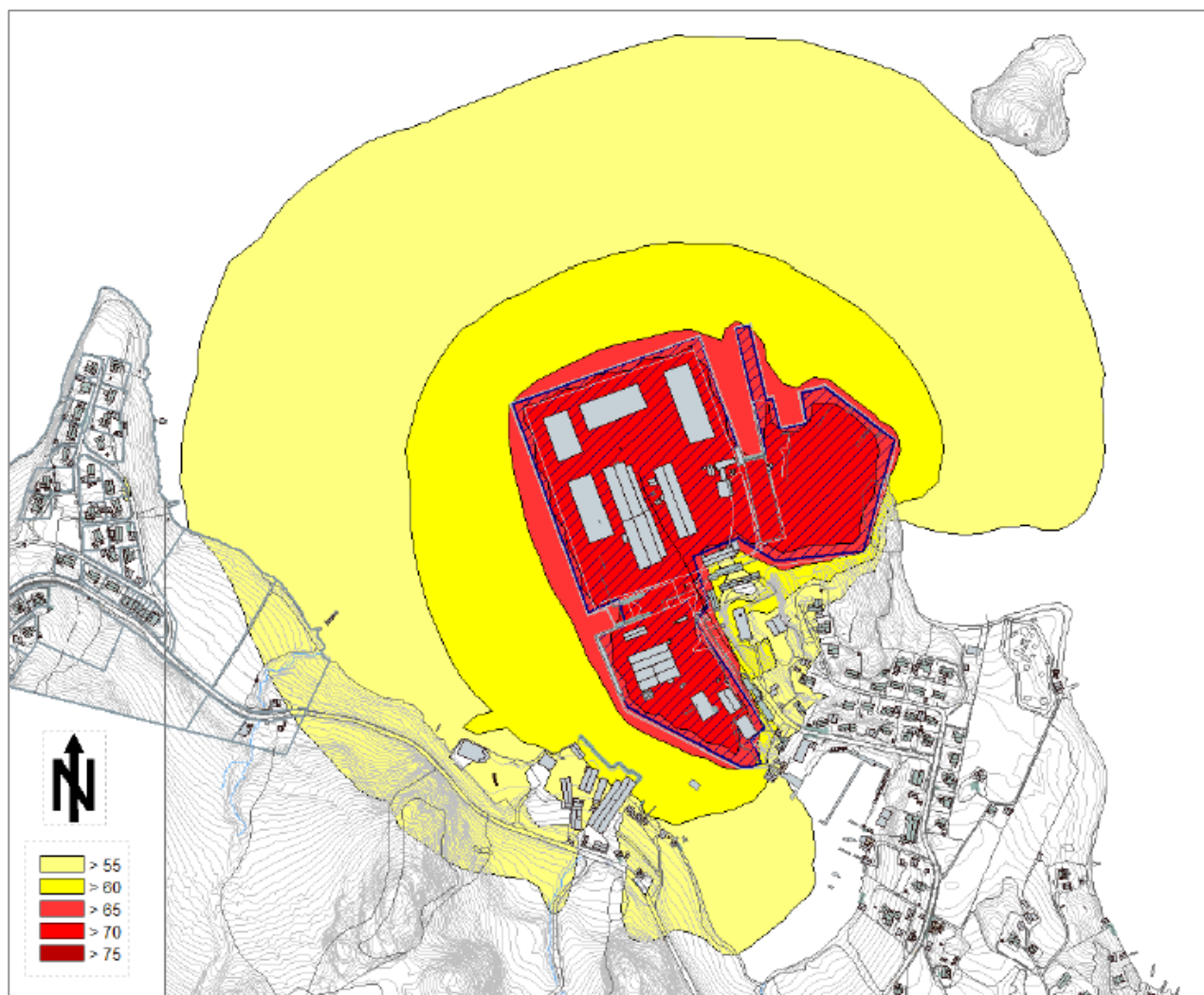
Figur 104: Beregna støysone i høgd +4 m for framtidig situasjon – med utbygging. Lydkjelde er markert med blå skravur. Brekke& Strand Akustikk AS.
