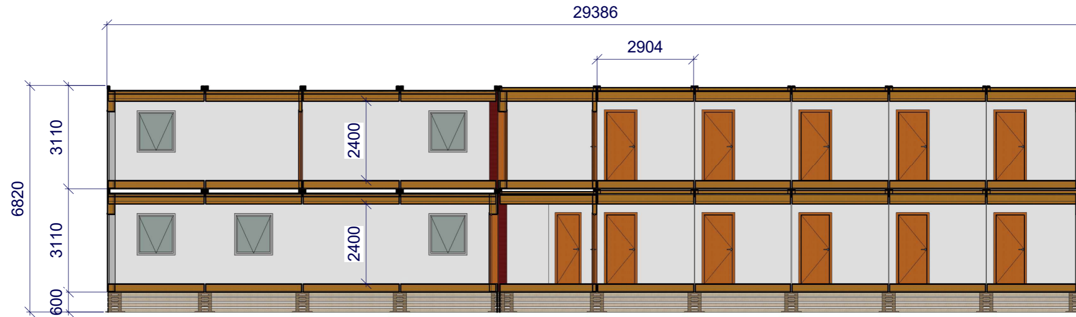
① Snitt - Boligrigg 1 : 100
