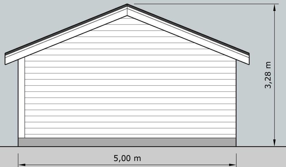
Fasade mot øst 1:50 A3
