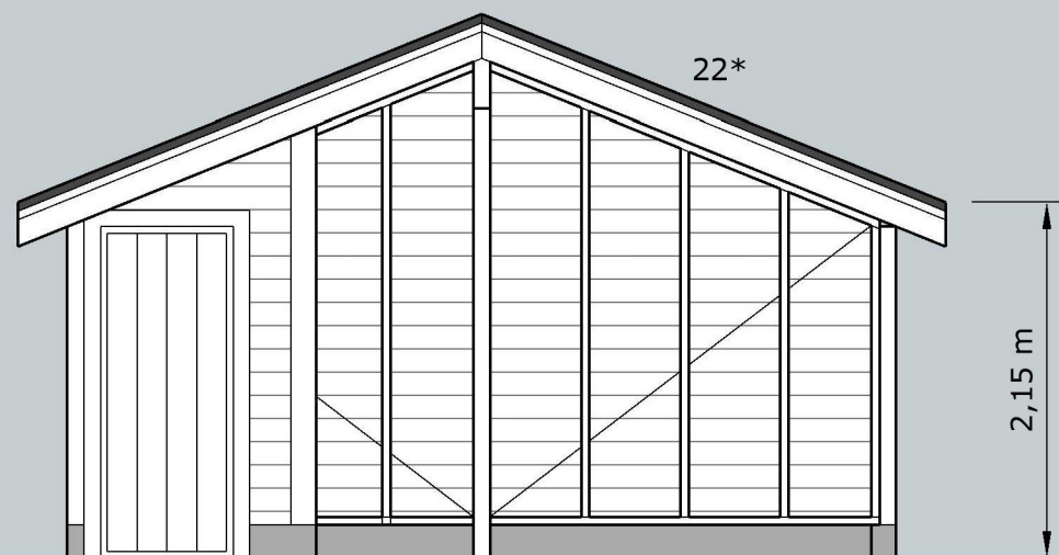
Fasade mot vest 1:50 A3
