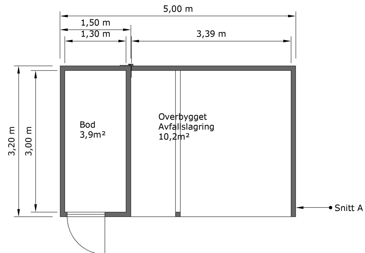
Plan 1:50 A3
