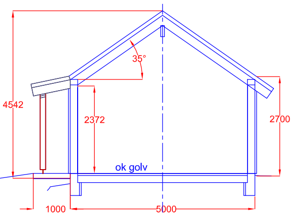
SNITT A - A
