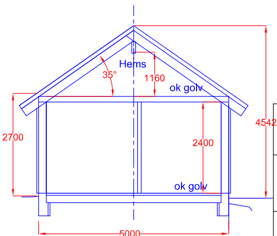
SNITT B - B
