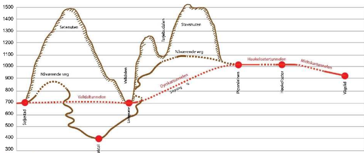
Figur 1, Illustrasjon av høgdeskilnad på eksisterande trase og ny trase
